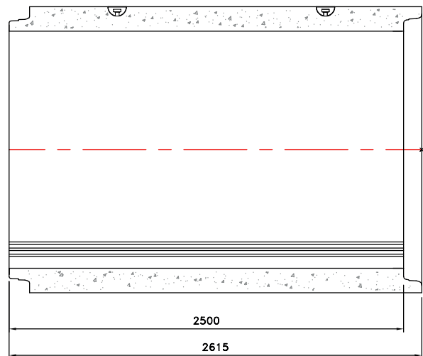
LONGITUDINAL SECTION
