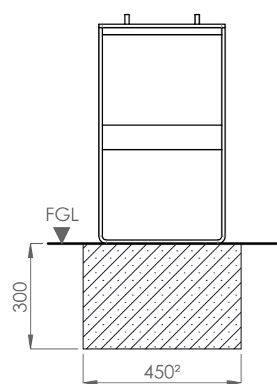
TYP FOUNDATION DETAIL SCALE 1 : 15
